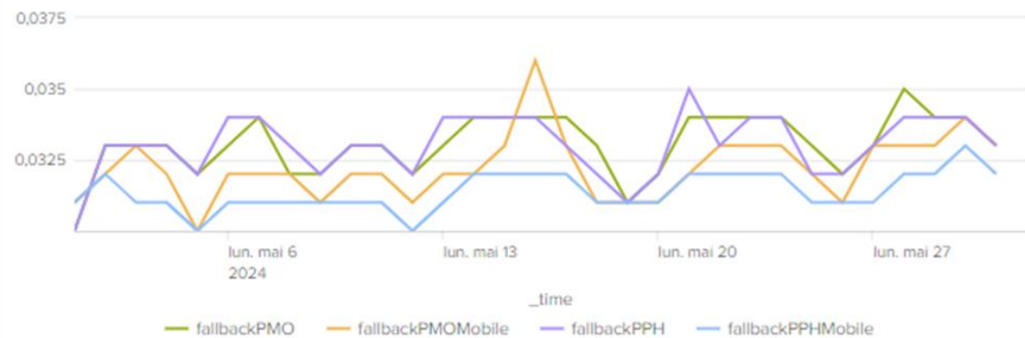
FALLBACK - Temps de réponse par endpoint
