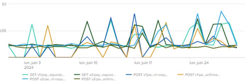
SANDBOX - Temps de réponse par endpoint CBPII
