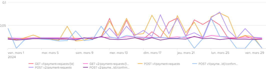
SANDBOX - Temps de réponse par endpoint CBPII
