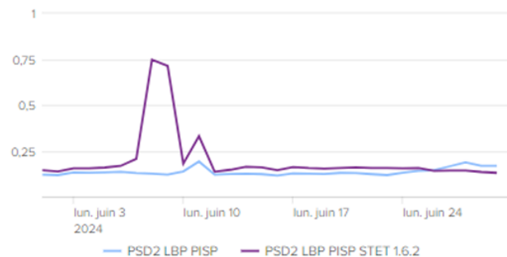
PISP - Temps de réponse POST /payment-requests
