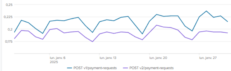
PISP - Temps de réponse GET /payment-requests/{id}
