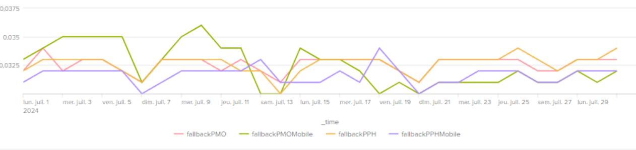
FALLBACK - Temps de réponse par endpoint
