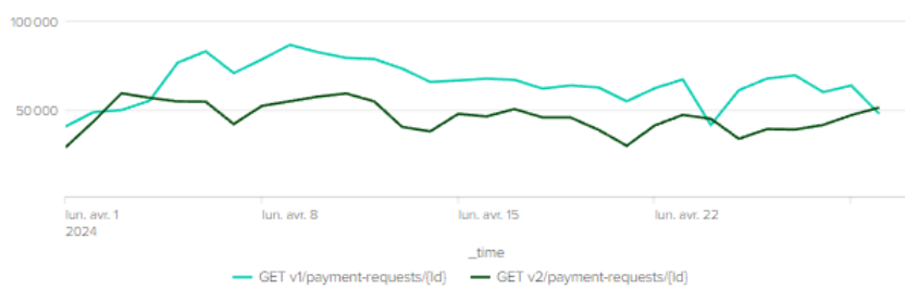
PISP - Nombre appels GET /payment-requests/{id}
