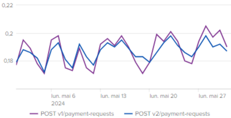
PISP - Temps de réponse POST /payment-requests
