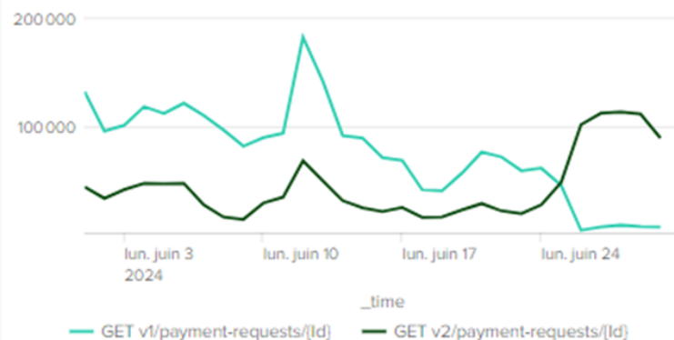
PISP - Nombre appels GET /payment-requests/{id}
