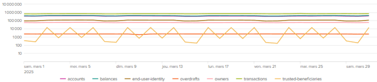
AISP - Nombre appels par endpoint
