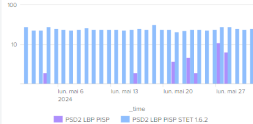
PISP - Nombre erreur 500 par API
