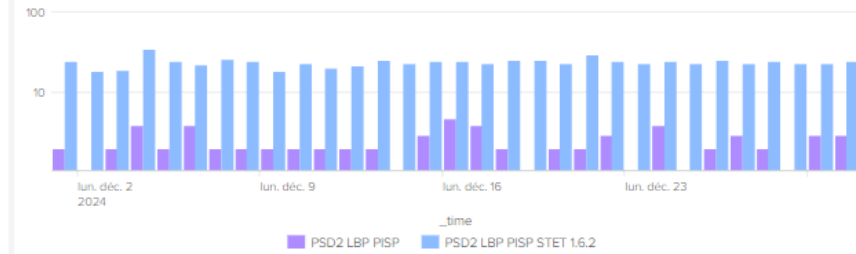
PISP - Nombre erreur 500 POST /payment-requests
