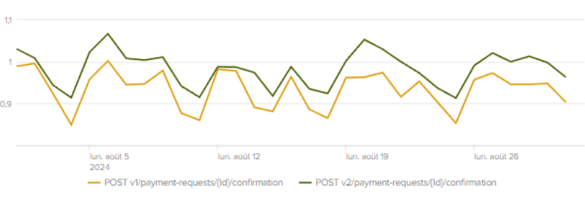
PISP - Temps de réponse PUT /payment-requests/{id}
