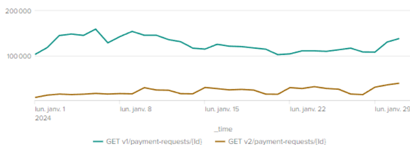
PISP - Nombre appels GET /payment-requests/{id}
