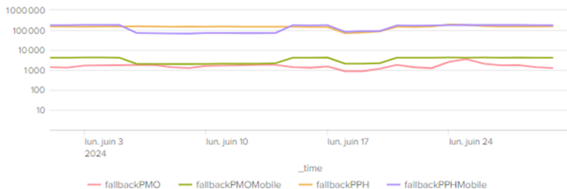
FALLBACK - Nombre erreur 500 par endpoint
