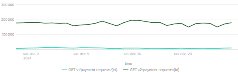
PISP - Nombre appels GET /payment-requests/{id}
