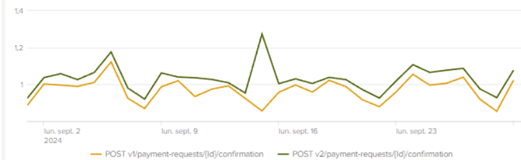
PISP - Temps de réponse POST /payment-requests/[id]/confirmation
