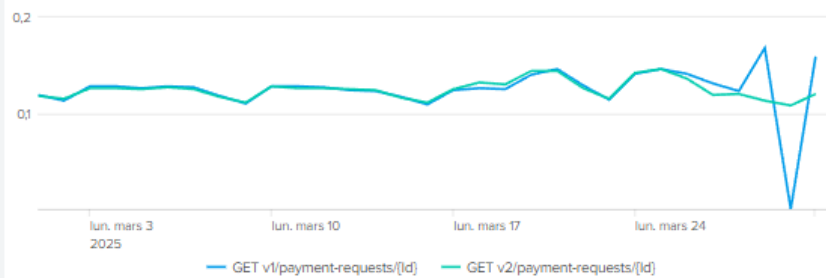
PISP - Temps de réponse GET /payment-requests/{id}
