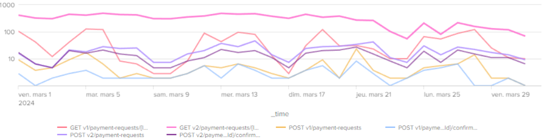
SANDBOX - Nombre appels par endpoint CBPII
