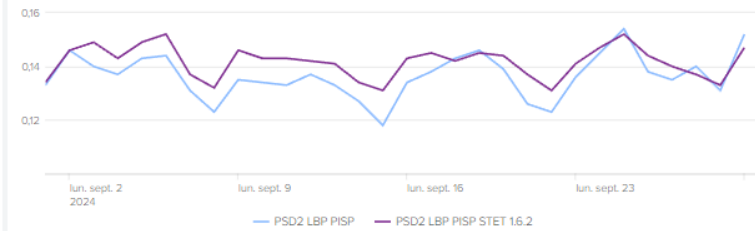
PISP - Temps de réponse POST /payment-requests
