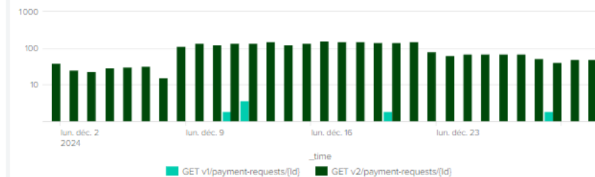
PISP - Nombre erreur 500 GET /payment-requests/{id}
