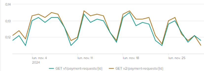
PISP - Temps de réponse GET /payment-requests/{id}
