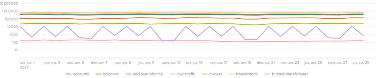
AISP - Nombre erreur 500 par endpoint
