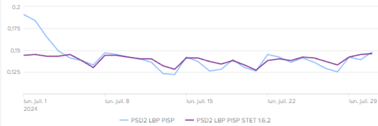
PISP - Temps de réponse POST /payment-requests
