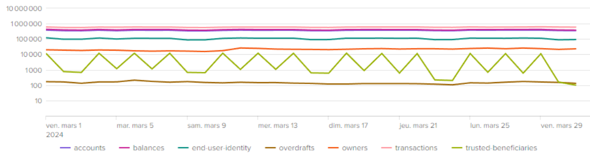
AISP - Nombre erreur 500 par endpoint
