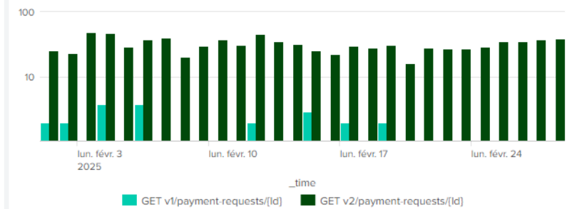
PISP - Nombre erreur 500 GET /payment-requests/{id}
