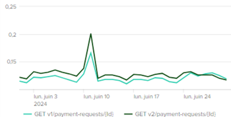
PISP - Temps de réponse GET /payment-requests/{id}
