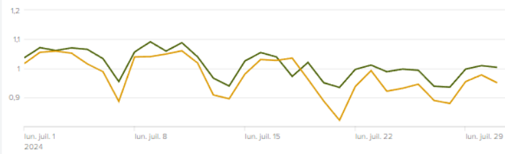
PISP - Temps de réponse POST /payment-requests/[id]/confirmation
